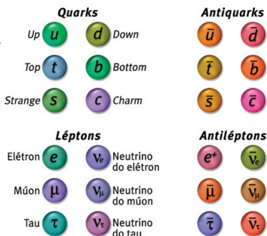
Figura 1. Quarks, léptons e suas respectivas antipartículas
