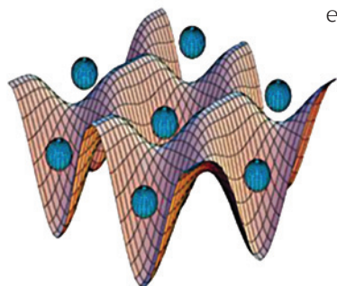
Átomos ocupando “vales” de uma rede cristalina óptica
